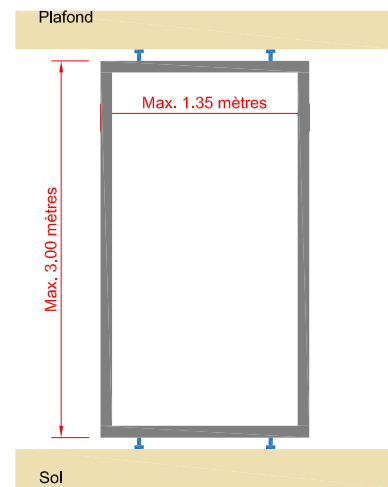
Pose avec des vérins à vis réglables de +/- 2 cm
