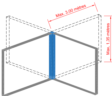
Modules de 2, 3 ou 4 panneaux fixés à 90° sur potelet central
